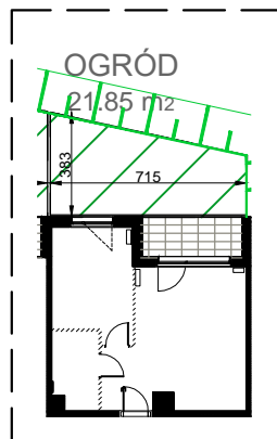
SCHEMAT MIESZKANIA WRAZ Z OGRÓDKIEM
