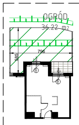
SCHEMAT MIESZKANIA WRAZ Z OGRÓDKIEM
